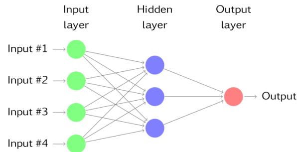
Fig 4 CNN
